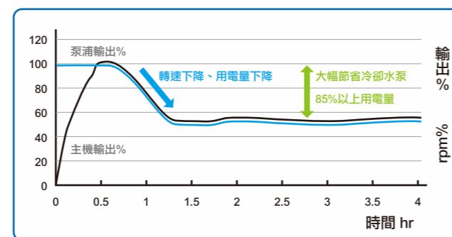
變流量控制 (Variable Flow Control)
